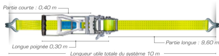
3 systèmes d'arrimage nécessaires* POWERTRUCK (LC 2500 daN) S_{TF} 800 daN
